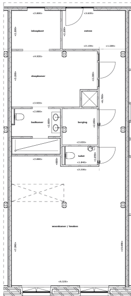
Plattegrond verdieping 02 1:50
